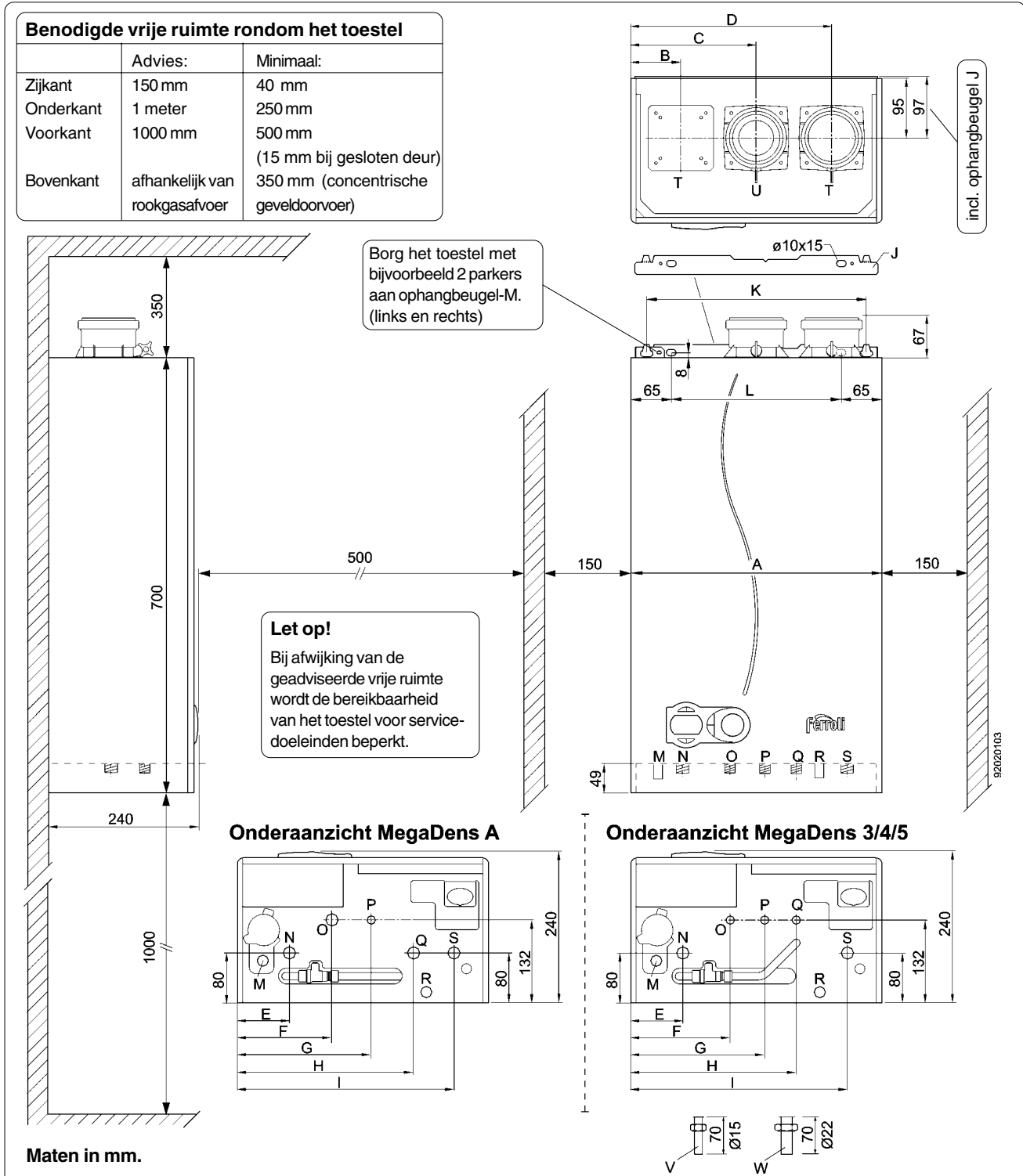
Figuur 10.1 Afmetingen en aansluitingen
